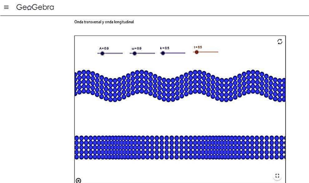
Figura 2. Simulador de tipos de ondas Fonte: Arquivo pessoal (2018).
