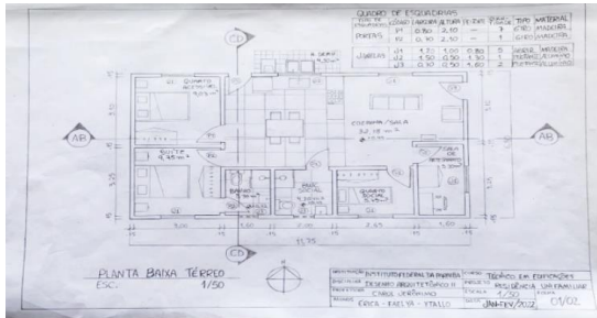
Fig.10 - Planta Baixa do projeto executada à mão com instrumentos entregue por uma das equipes de estudantes da turma.
