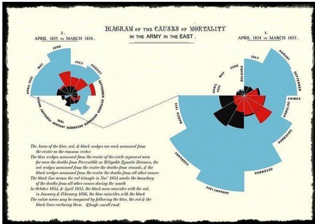
Figura 1: Diagrama Rosa
