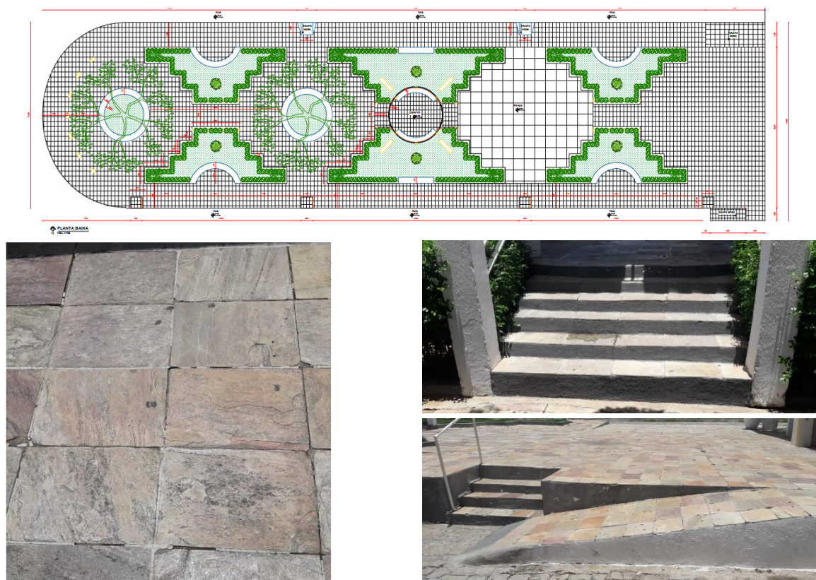
Figura 1 – Praça pública municipal: a) Planta baixa; b) Piso em pedra lapidada; c) Escada de acesso ao coreto; d) Rampa e escada de acesso à praça.
