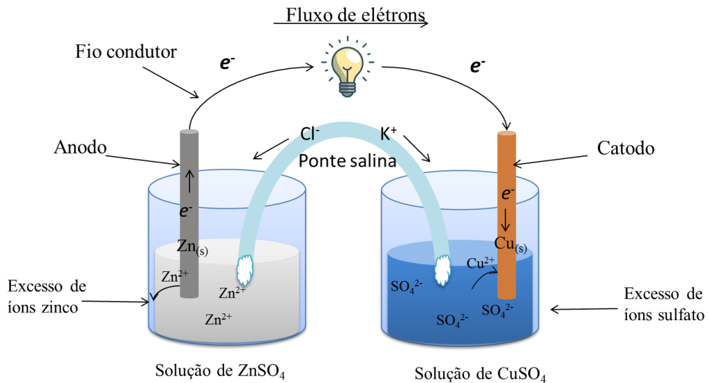
Figura 3: Esquema eletroquímico da pilha de Daniell. FONTE: Adaptado de Chang e Goldsby, 2013.
