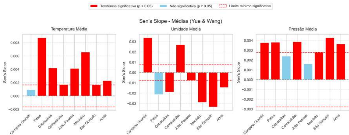
Figura 11: Tendências das variáveis médias por cidade
