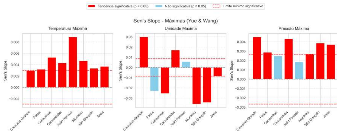
Figura 10: Tendências das variáveis máximas por cidade
