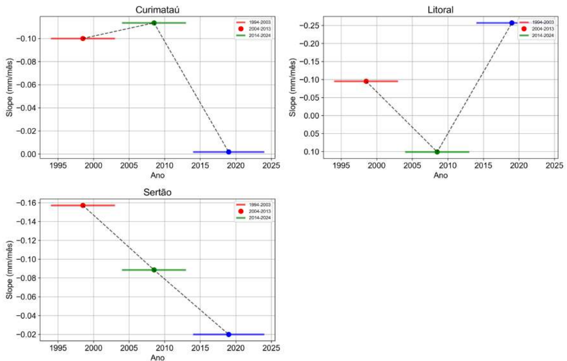
Figura 6: Sen's Slope por faixa de anos
