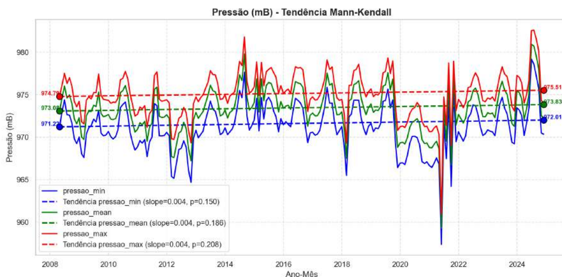
Figura 7: Variação da pressão atmosférica ao longo do tempo
