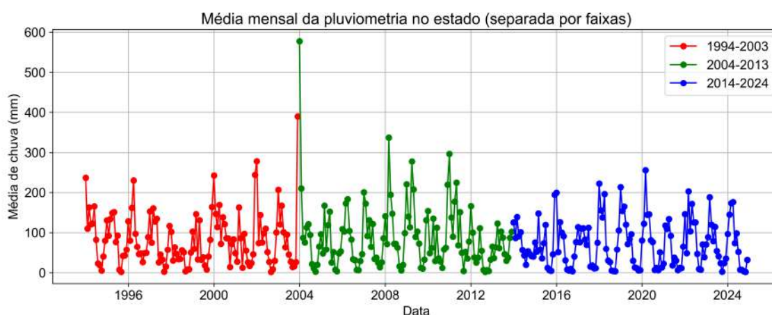
Figura 1: Média mensal de chuvas no período de 1994 a 2024
