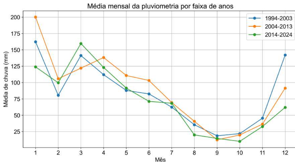
Figura 2: Média mensal da pluviometria por faixa de anos
