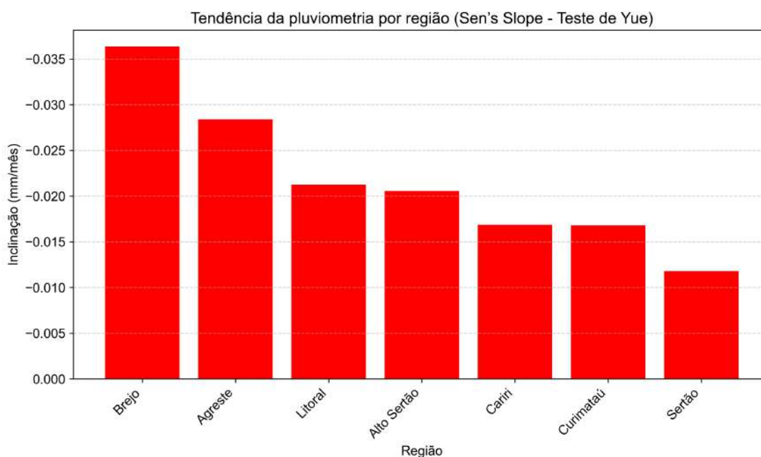
Figura 5: Tendência da pluviometria por região (Sen's Slope - Teste de Yue)
