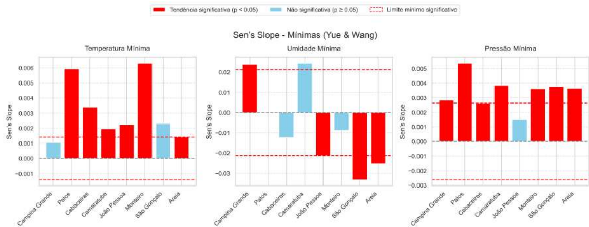
Figura 12: Tendências das variáveis mínimas por cidade
