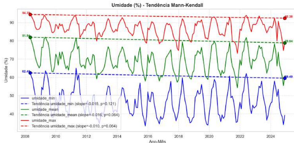
Figura 9: Variação da umidade ao longo do tempo
