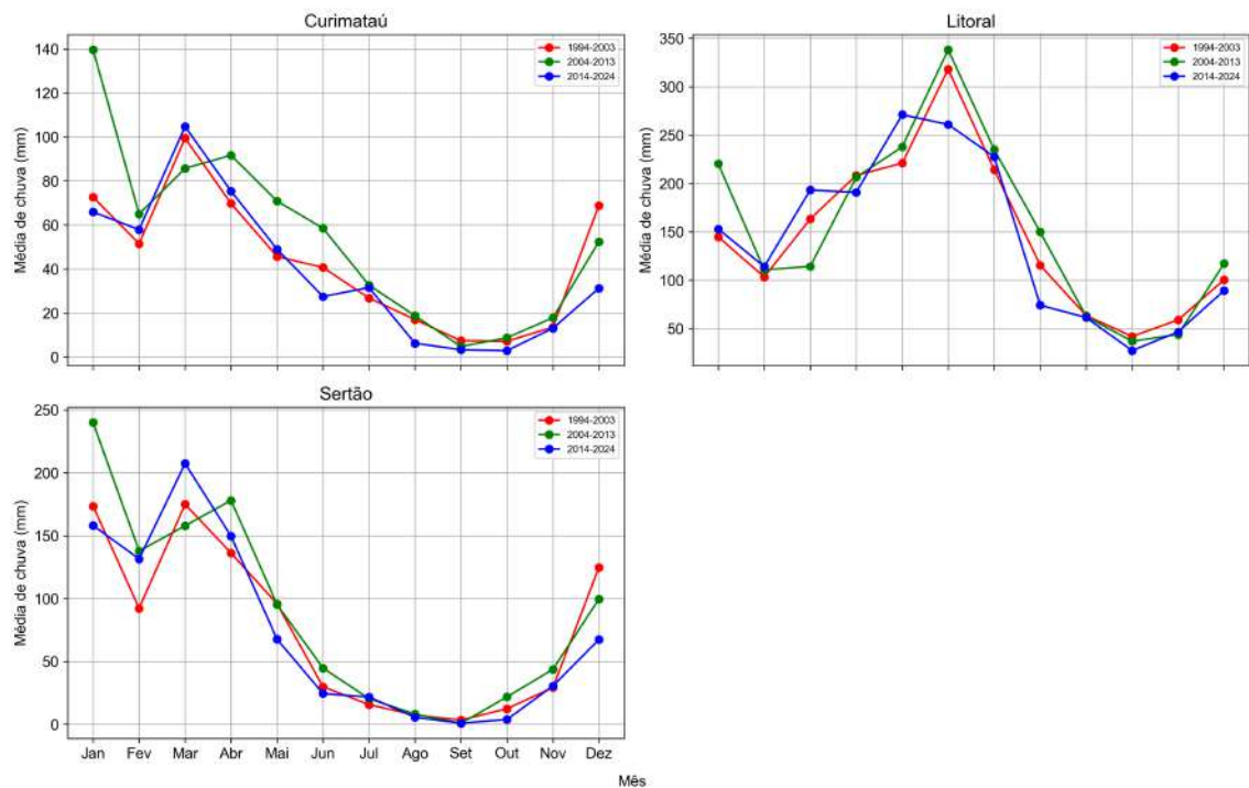
Figura 4: Chuva mensal por região (por faixa de anos)
