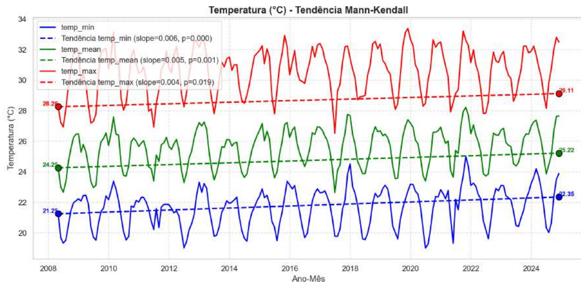
Figura 8: Variação da temperatura ao longo do tempo
