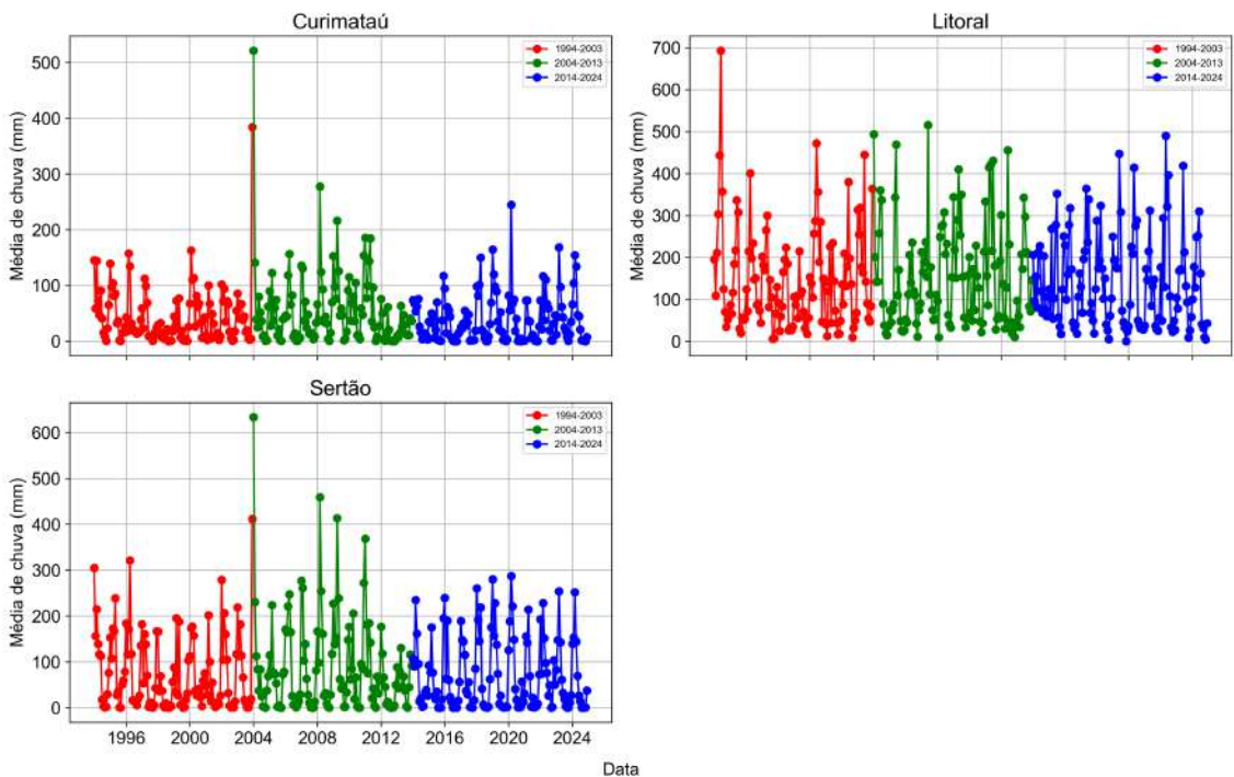
Figura 3: Chuva mensal por região (por faixa de anos)
